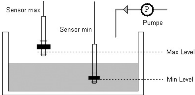
Fig. 3: aquaniveau con dos flotadores de encendido
