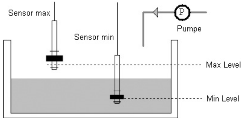
Fig. 3: aquaniveau con due interruttori a galleggiante
