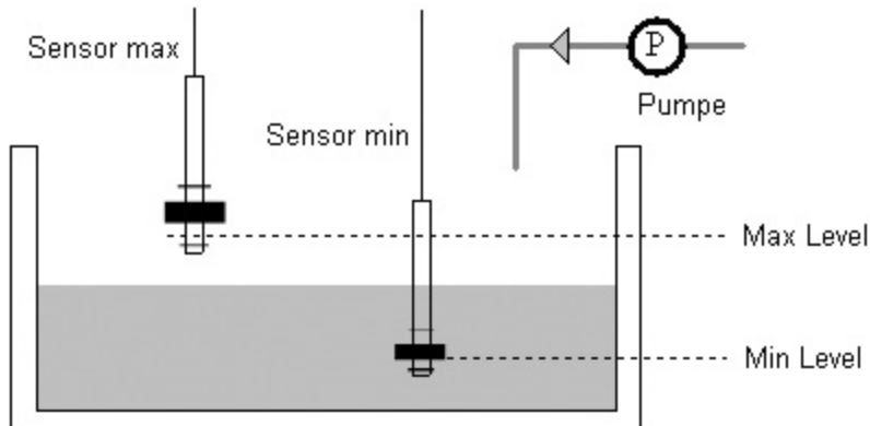
Abb. 3: aquaniveau mit 2 Schwimmerschaltern
